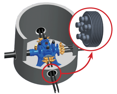
Stikkledningskum med Basal Manifold pakning F 911-5
